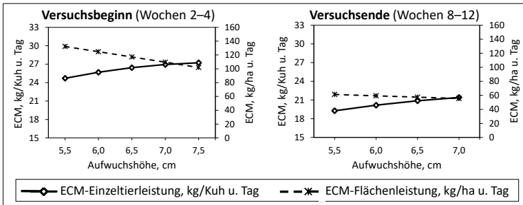
Abb. 1. ECM-Einzeltier- und ECM-Flächenleistungen (kg je Tag) bei unterschiedlicher Weide-Aufwuchshöhe zu Versuchsbeginn (Versuchswochen 2-4) bzw. zu Versuchsende (Versuchswochen 8-12)
