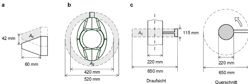
Abbildung 1: Draufsicht auf ein a. Doppelmessermähwerk und b. Scheibenmähwerk sowie Draufsicht und Querschnitt eines c. Schlegelmähwerks mit der in Grau markierten Fläche A_E , die von einem Messer während eines Hubs beziehungsweise einer Umdrehung beeinflusst wird.
